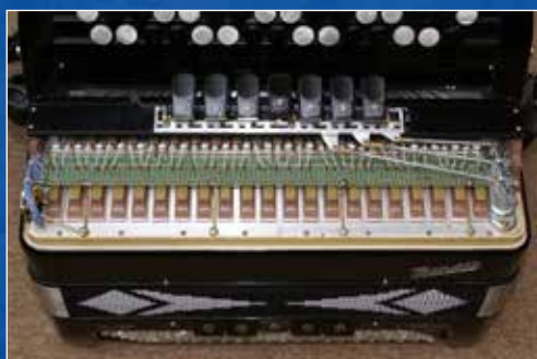
Kontaktbrygga på diskantsidan
